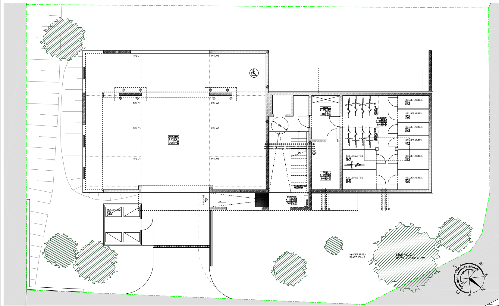
KELLERGESCHOSS M 1: 50
